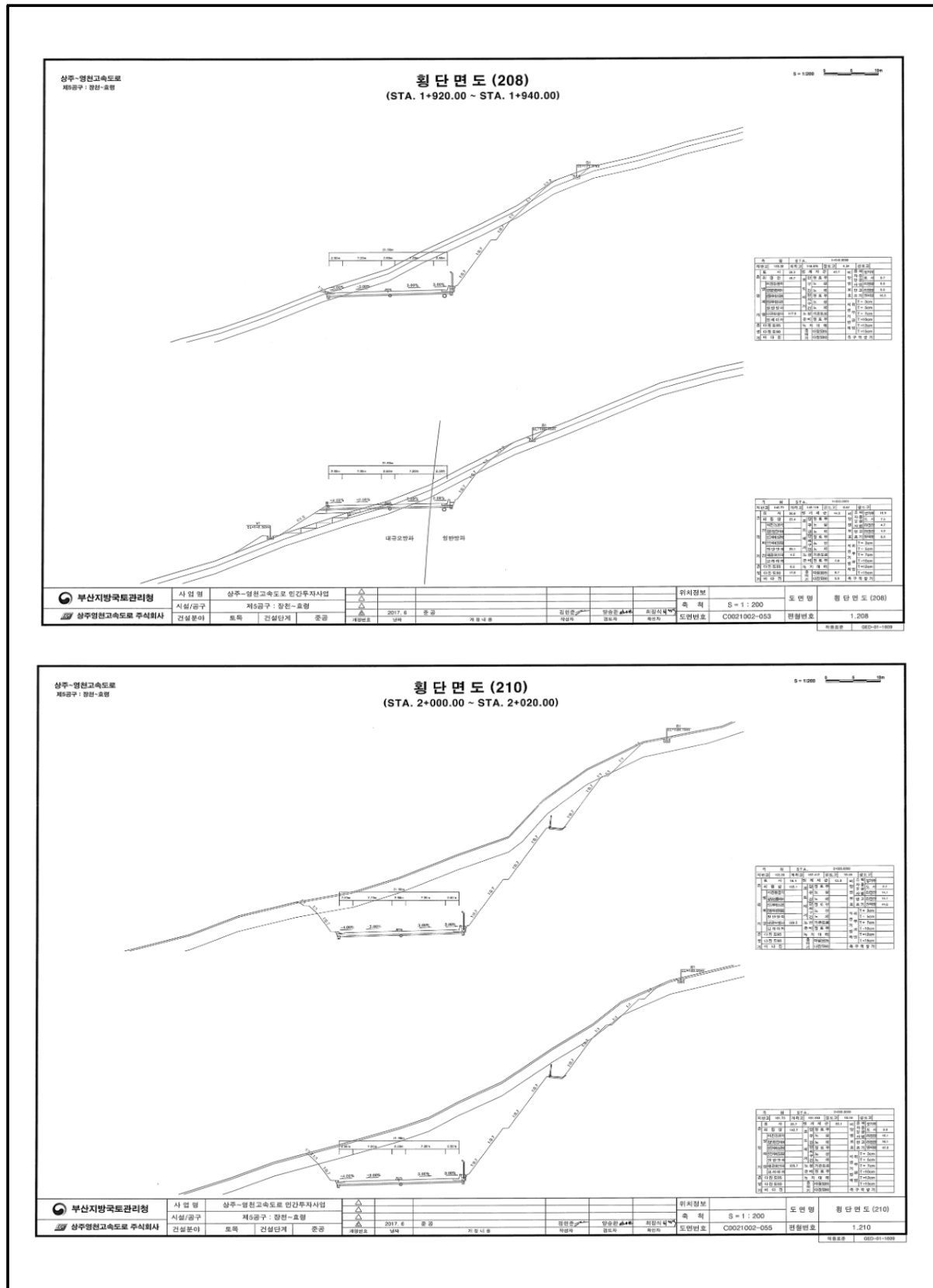
【그림 34.4】 표준횡단면도
